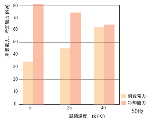
凝縮温度別消費電力・冷却能力推移グラフ ※三菱電機製スクロール二段圧縮式冷凍機MSW-SP650A-tk（定格65 kW） 蒸発温度to=-45°Cの \eta_{max} システム専用能力表より
